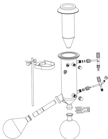
G5 / G5B - chladič pro nízkovroucí látky
