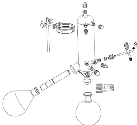
G6 / G6B - vertikální chladič pro destilaci s refluxem
