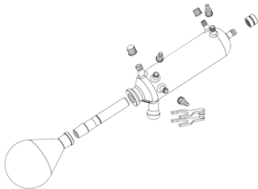
G5 / G5B - chladič pro nízkovroucí látky
