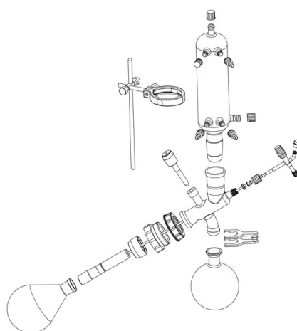
G6 / G6B - vertikální chladič pro destilaci s refluxem
